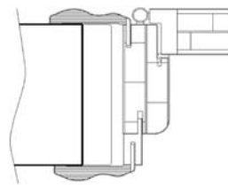
Sezione prolungamento - tipo A Section extension type "A"
