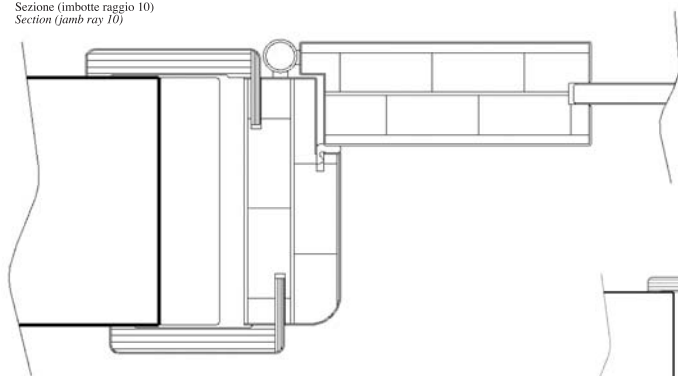
Sezione imbotte vano passaggio Section jamb vain passage
