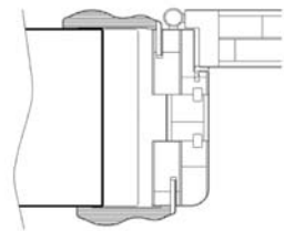
Sezione prolungamento - tipo B Section extension type "B"
