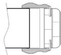
Sezione imbotte vano passaggio Section jamb vain passage
