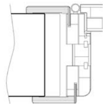
Sezione prolungamento - tipo B Section extension type "B"
