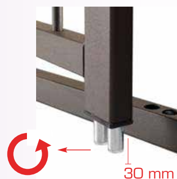
Dettaglio puntali in acciaio, uno dei due ha la caratteristica di essere ROTANTE/ANTITAGLIO
