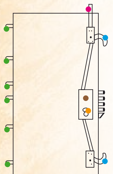
Figura 2: Limitatore di apertura laterale
